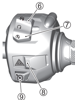
RECHTE LENKERARMATUR
